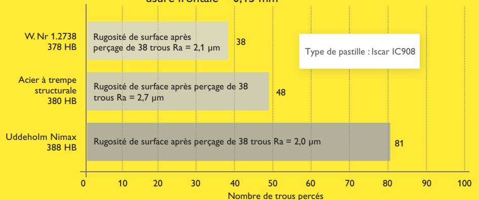
Figure 2 - Comparaison : nombre de trous percés avant usure frontale = 0,15 mm
